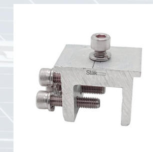
STAK-G-50 G-CLIP PARA TEJA TRASLAPADA
